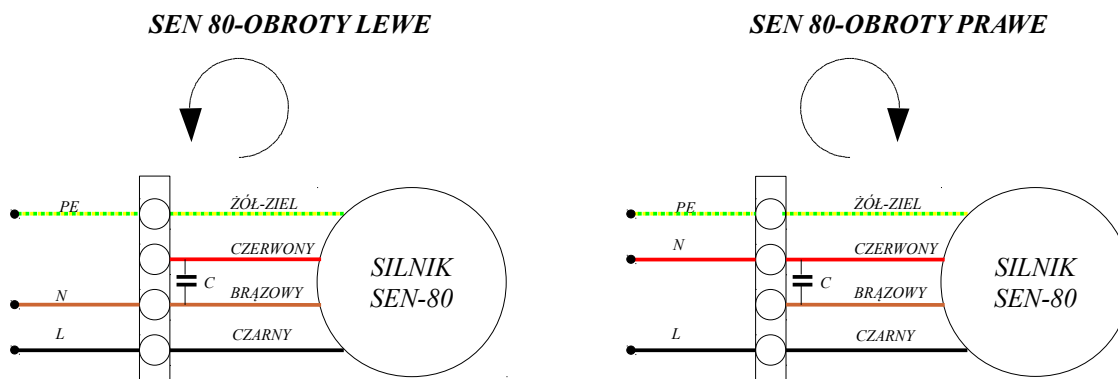
Rys.4.Podłączenie w wersji standard.
